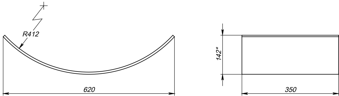
Поз.3 (Ложемент)
